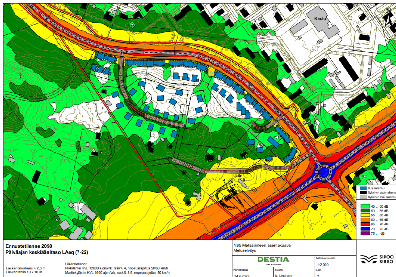
Metsärinteen meluselvitys, päiväajan keskiäänitaso (Destia, 2023). Bullerutredning, Skogsliden, medelljudnivå dagtid (Destia, 2023).
