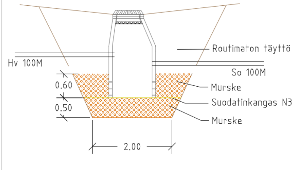
Kuva 12. Imeytyskaivon tyypipikuva.
