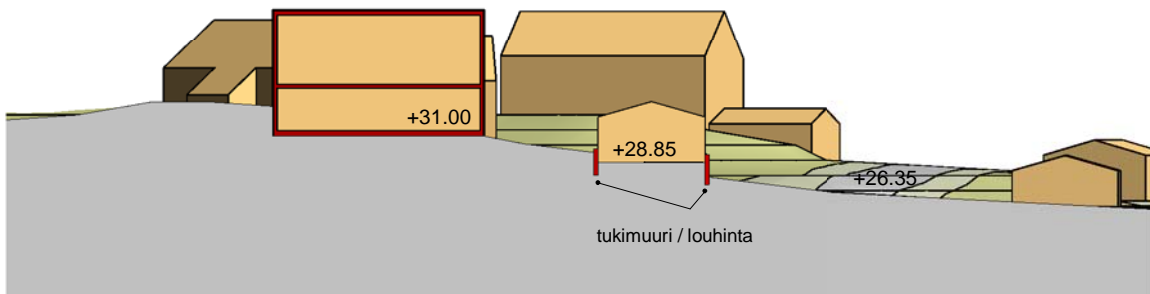
2. Kortteli 86 tontti 2, leikkaus 1 : 500
