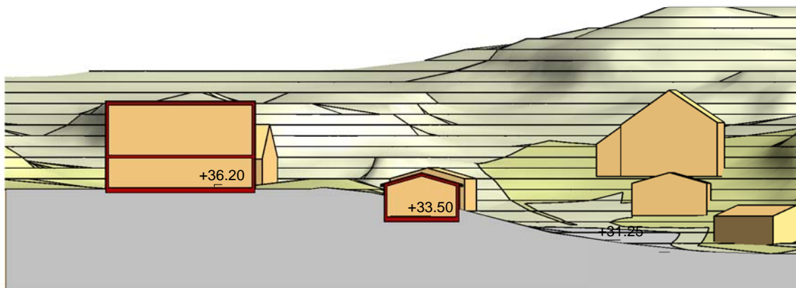
2. Kortteli 75 tontti 5, leikkaus 1 : 500
