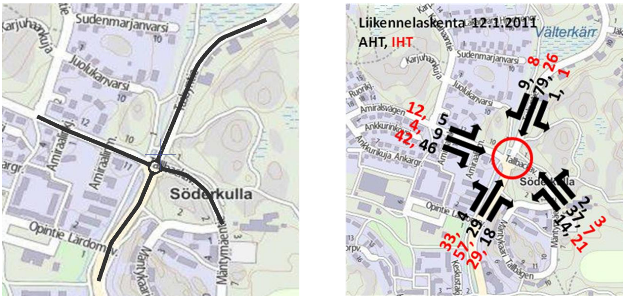
Kuva 1. Tarkasteltava kiertoliittymä ja keskiviikkona 12.1.2011 tehdyn liikennelaskennan tulos.
