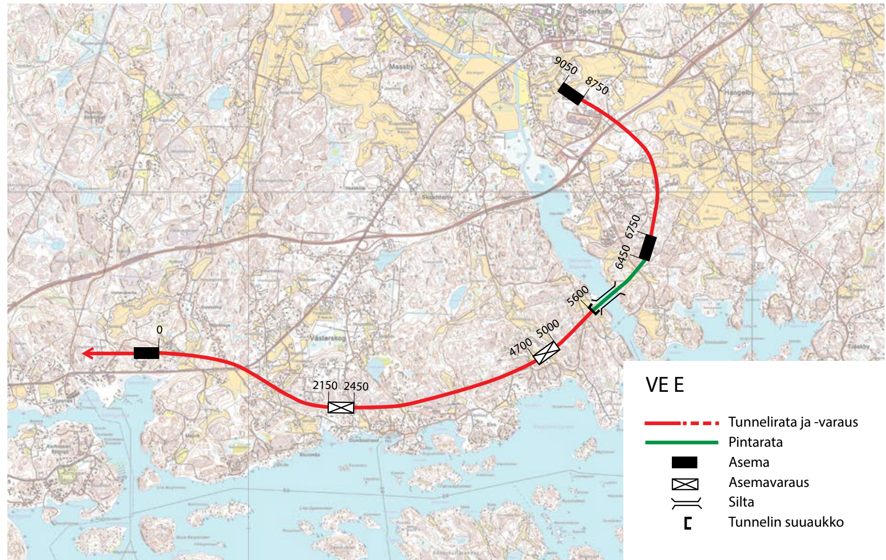
Kuva 29. Vaihtoehtoon E ensivaiheen suunnitelma
