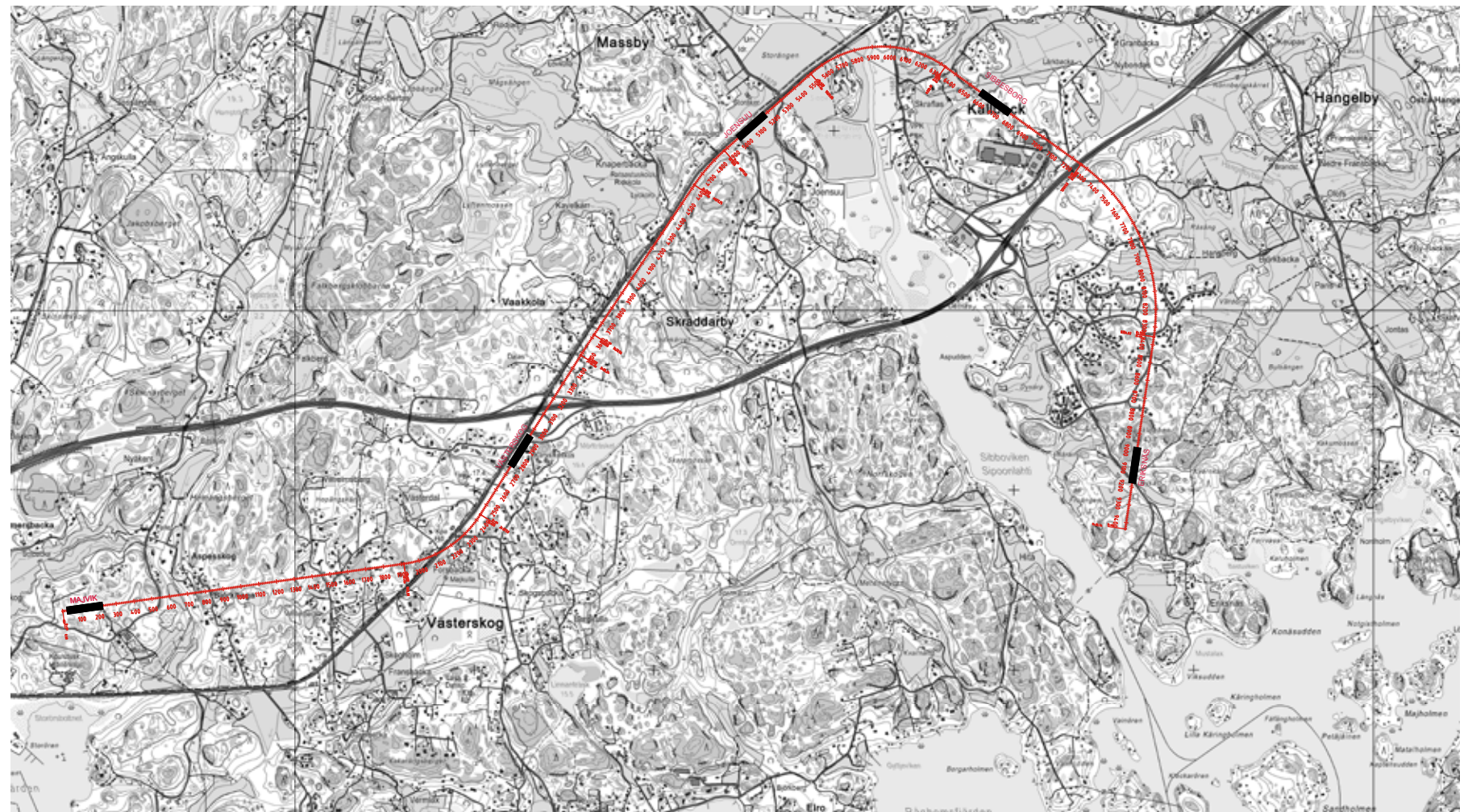
Kuva 25. Vaihtoehdon B metrolinjas nykyisessä maastossa
