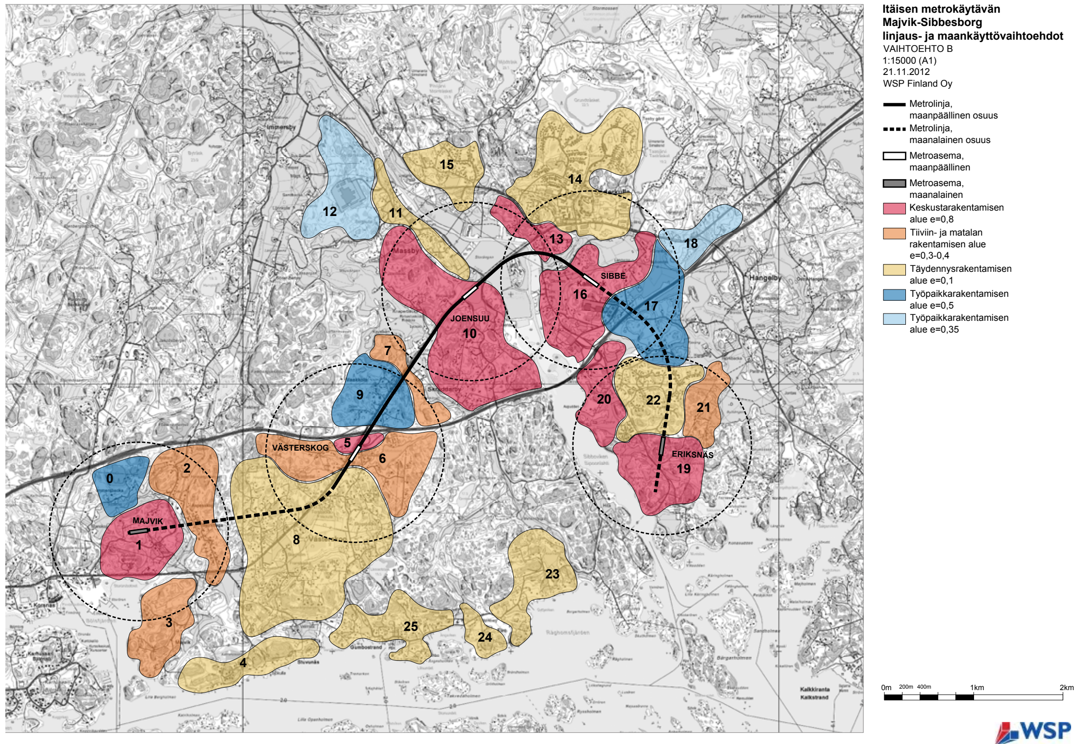
Kuva 26. Vaihtoehdon B metrolinjaus ja rakennemalli
