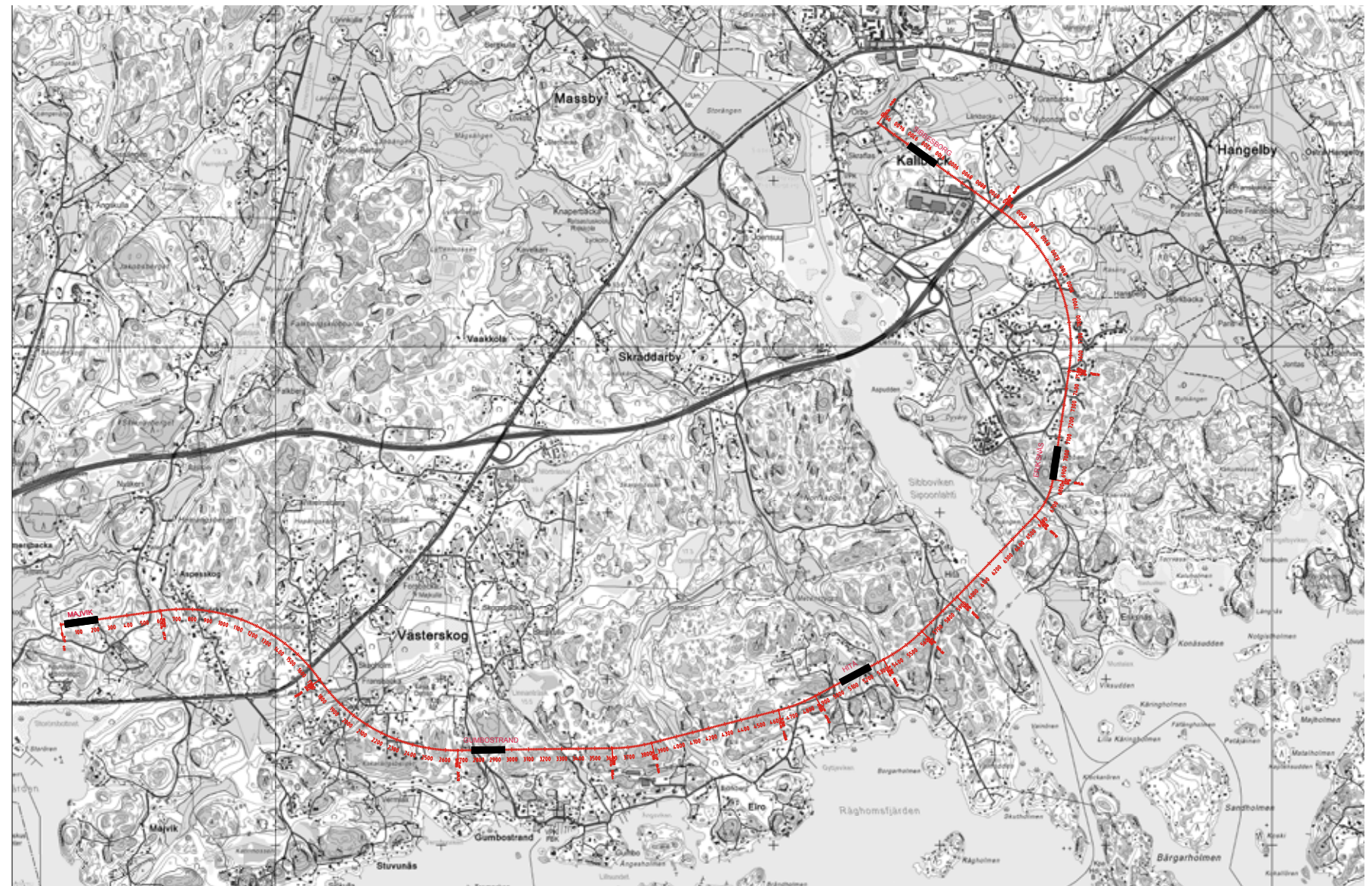
SIIPON METROLINJAUSVAIHTOEHDOT, LINJAUS E (suunnitteluvaihe 1) WSP Finland Oy 14.12.2012 mk 1:10000 (A1)
