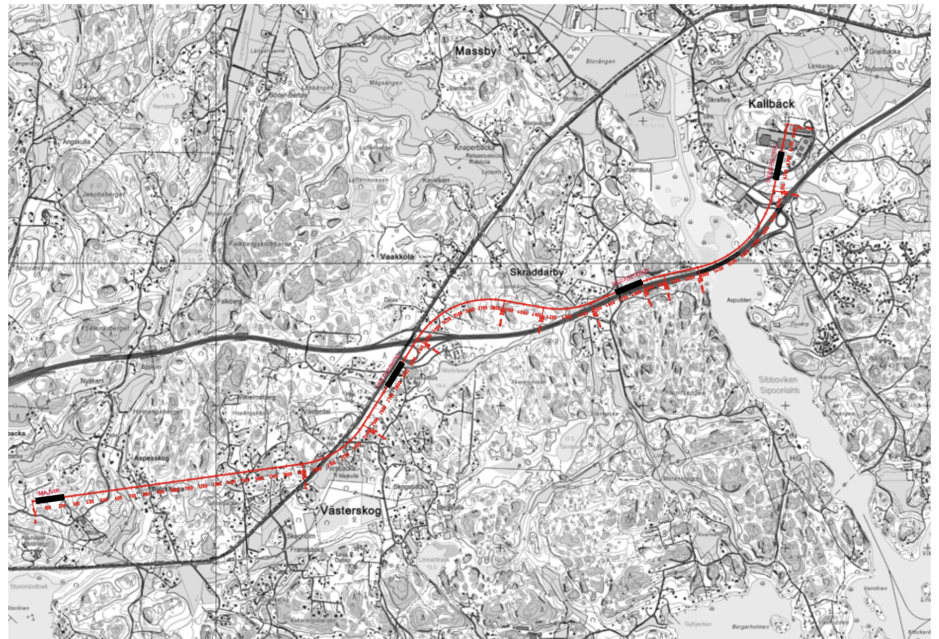
Kuva 39. AC – metrolinjaus ja asemien sijainti
