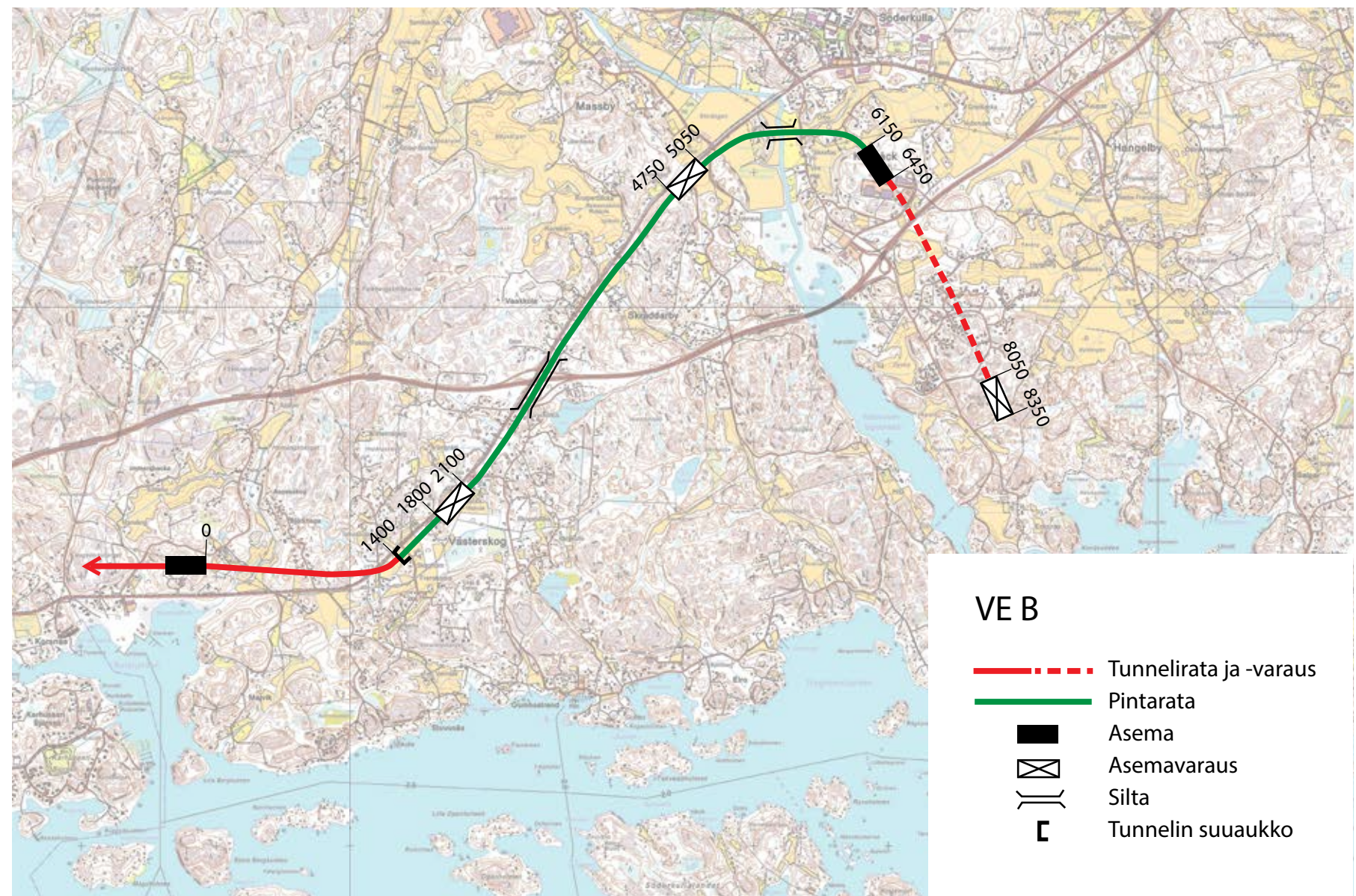
Kuva 23. Vaihtoehtoon B ensimmäinen versio linjauksesta
