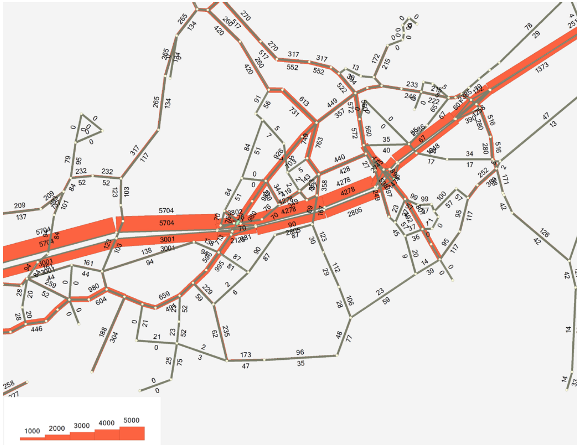
Kuva 53. Henkilöautoverkon kuormitus, kun moottoritiellä lisäkaistat [ajoneuvoa/aamuhuipputunti].
