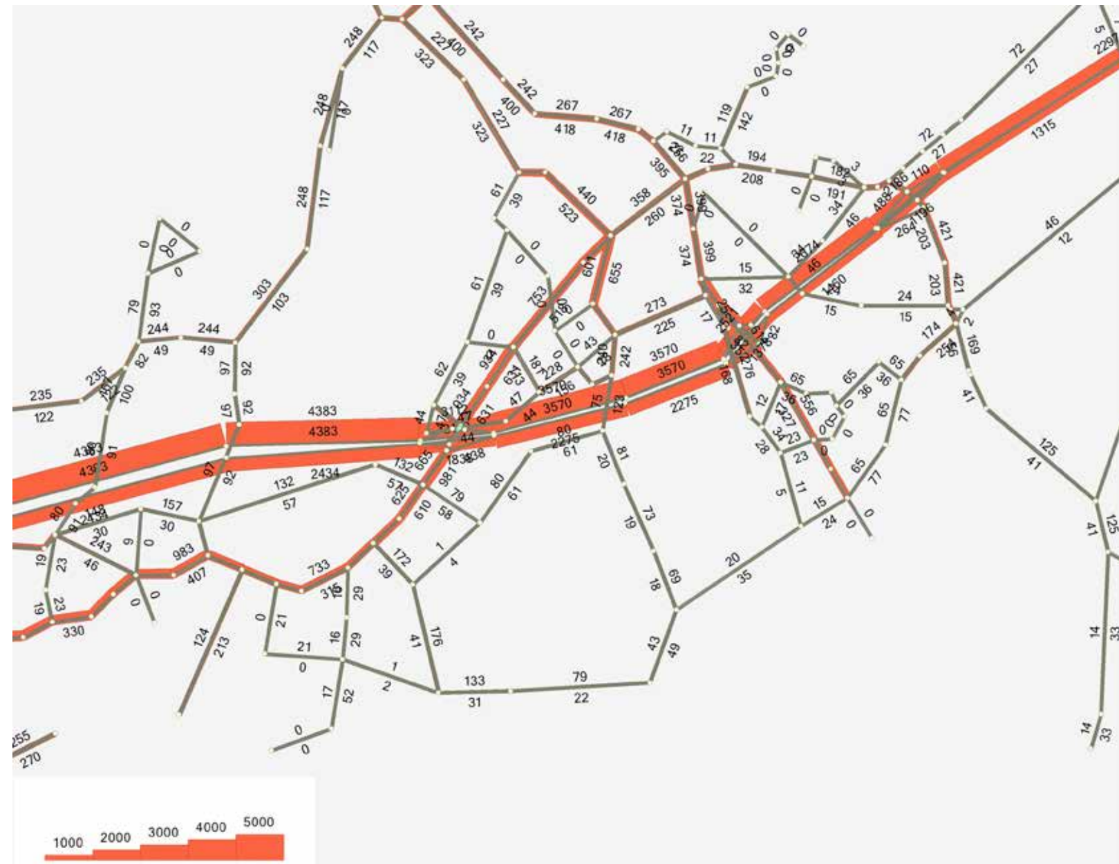
Kuva 55. Henkilöautoverkon kuormitus, kun maankäytön volyymi 70 % tavoitellusta [ajoneuvoa/aamuhuipputunti].
