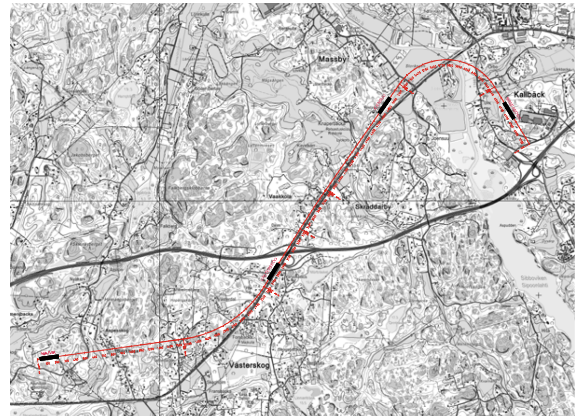
Kuva 45. B – metrolinjaus ja aseman sijainti
