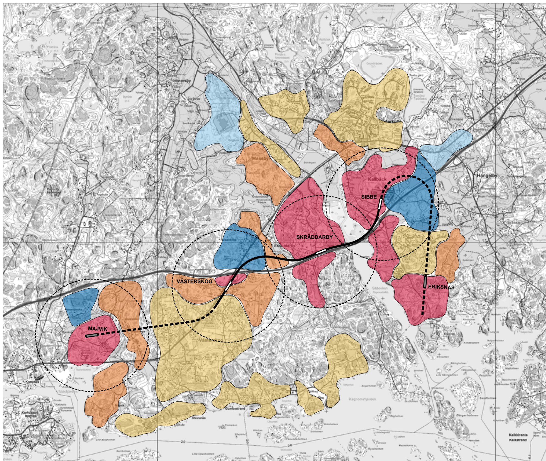
Kuva 20. Vaihtoehdon AC metrolinjaus ja rakennemalli
