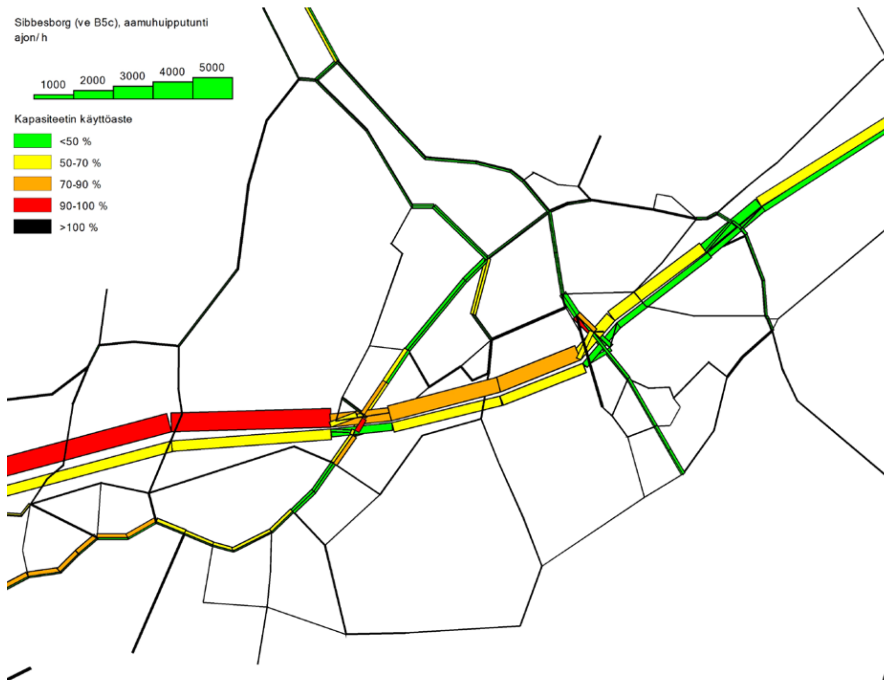
Kuva 56. Henkilöautoverkon kapasiteetin käyttöaste tarkastelualueella aamuhuipputuntina, kun maankäytön volyymi 70 % tavoitellusta.
