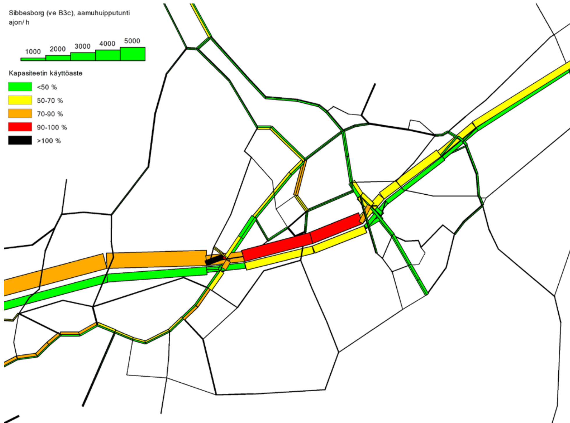
Kuva 54. Henkilöautoverkon kapasiteetin käyttöaste tarkastelualueella aamuhuipputuntina, kun moottoritiellä lisäkaistat
