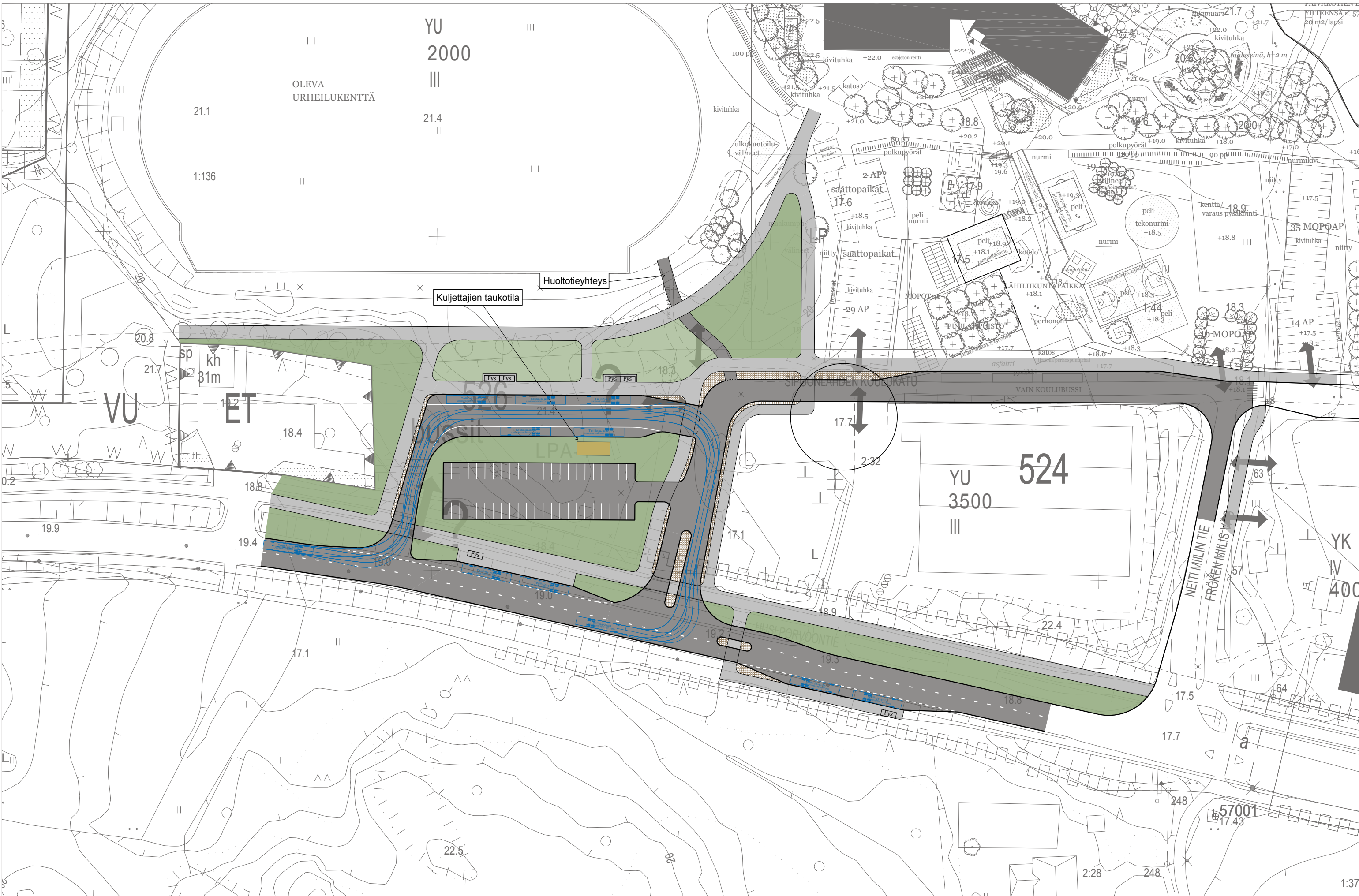
Sipoonlahden koulu Bussiterminaalin periaateratkaisu, mk 1:1000 (A3) 1.2.2017 WSP
