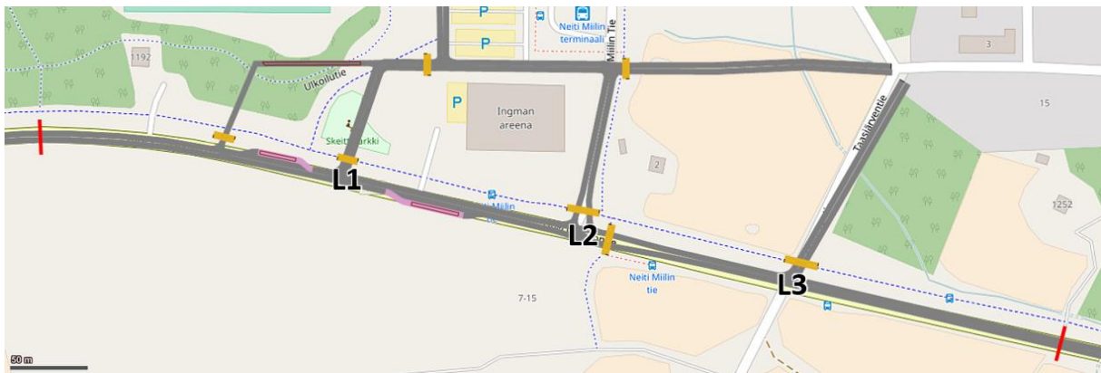
Kuva 27. Liikenteen toimivuuden mittauspisteet: liittymänumerot ja matka-aika.
