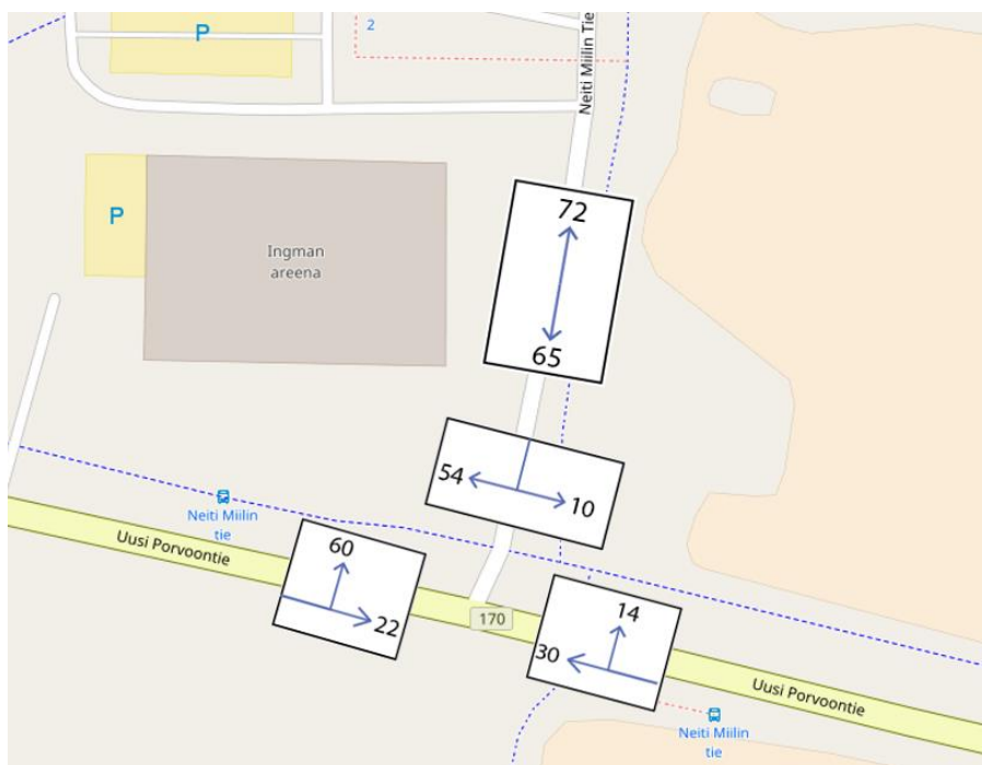
Kuva 3. Automäärät huippuvartina klo 8.30–8.45 Neiti Miilin Tien ja Uuden Porvoontien liittymässä sekä Neiti Miilin Tien poikkileikkaukskohdassa.
