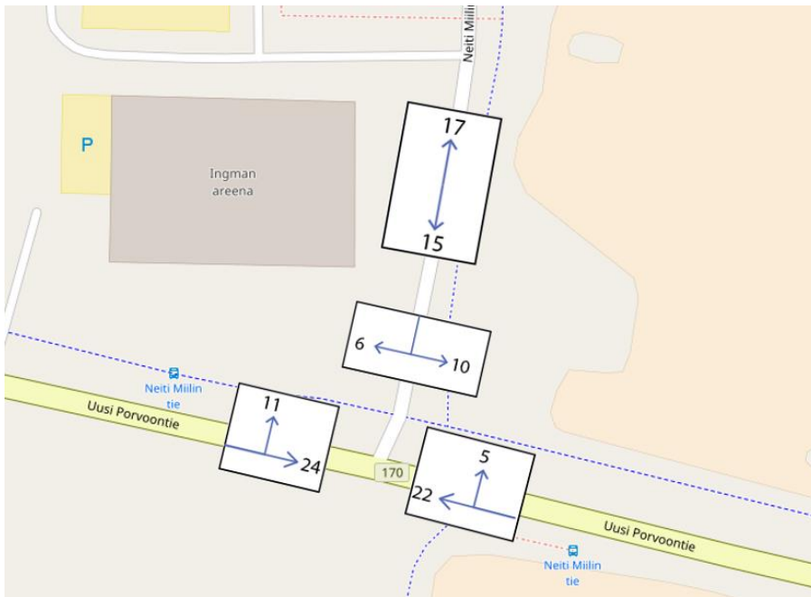
Kuva 4. Automäärät klo 8.45–9.00 Neiti Miilin Tien ja Uuden Porvoontien liittymässä sekä Neiti Miilin Tien poikkileikkauskohdassa.
