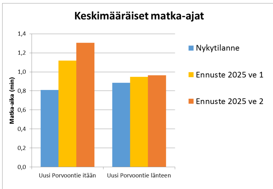
Kuva 29. Aamuhuipputunnin keskimääräiset matka-ajat Uudella Porvoontiellä idän ja lännen suuntaan nykytilanteessa ja vuoden 2025 ennustetilanteissa.
